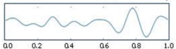
Fig. 4. Theta wave
