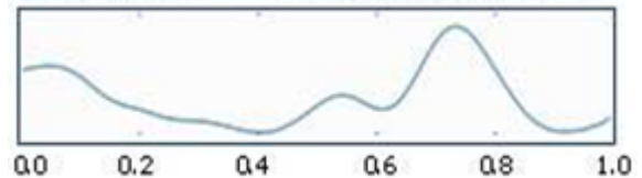
Fig. 3. Delta wave
